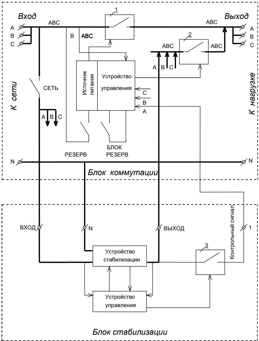
Рис. 4.1 Структурная схема стабилизатора
